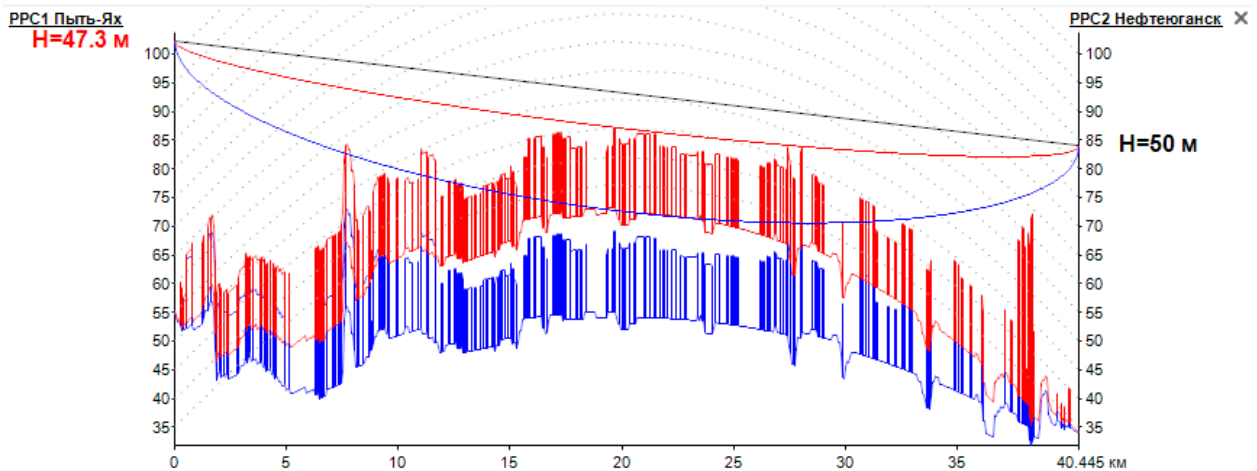
Рисунок 15. Изображение продольного профиля при расчете высот антенн
